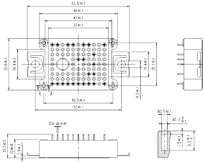
断面 A-A (1.5 : 1) SECTION A-A
