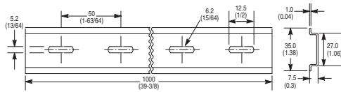
DIN Rail
