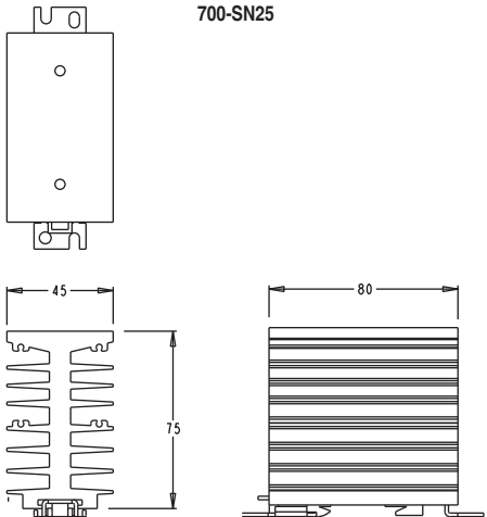
700-SN25
