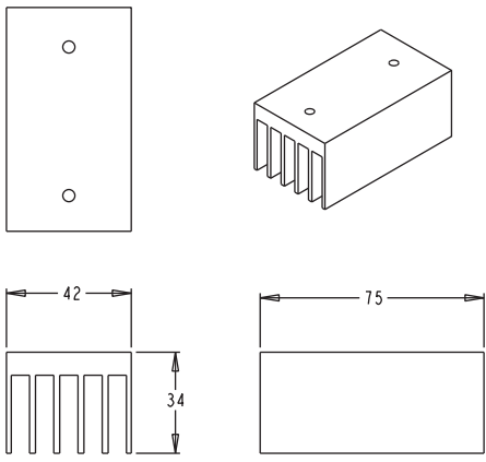
700-SN10
